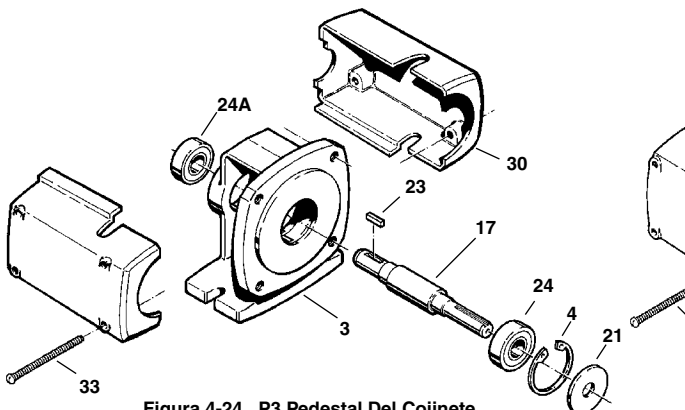
Figura 4-24 P3 Pedestal Del Cojinete
